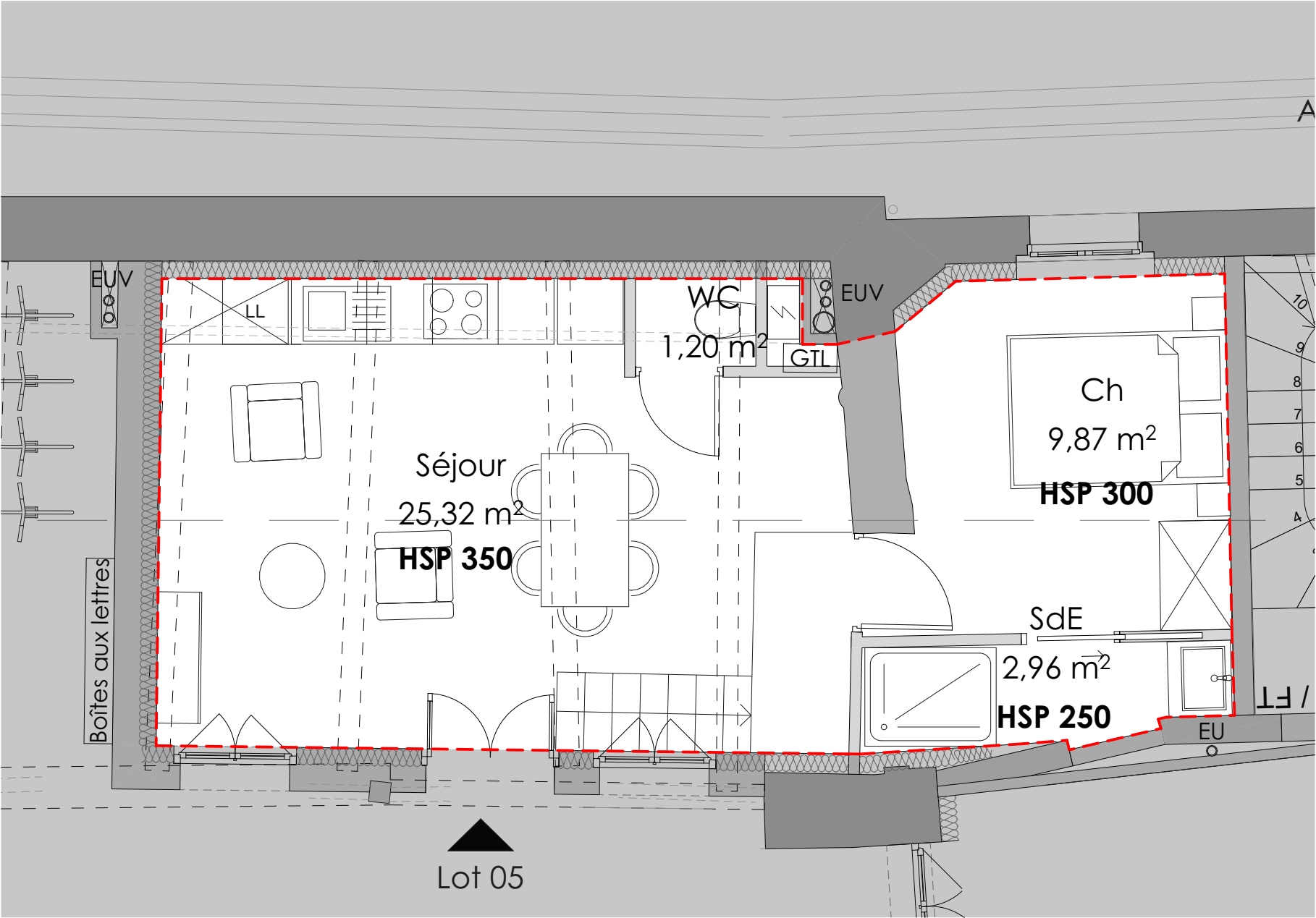
Plan RdC
