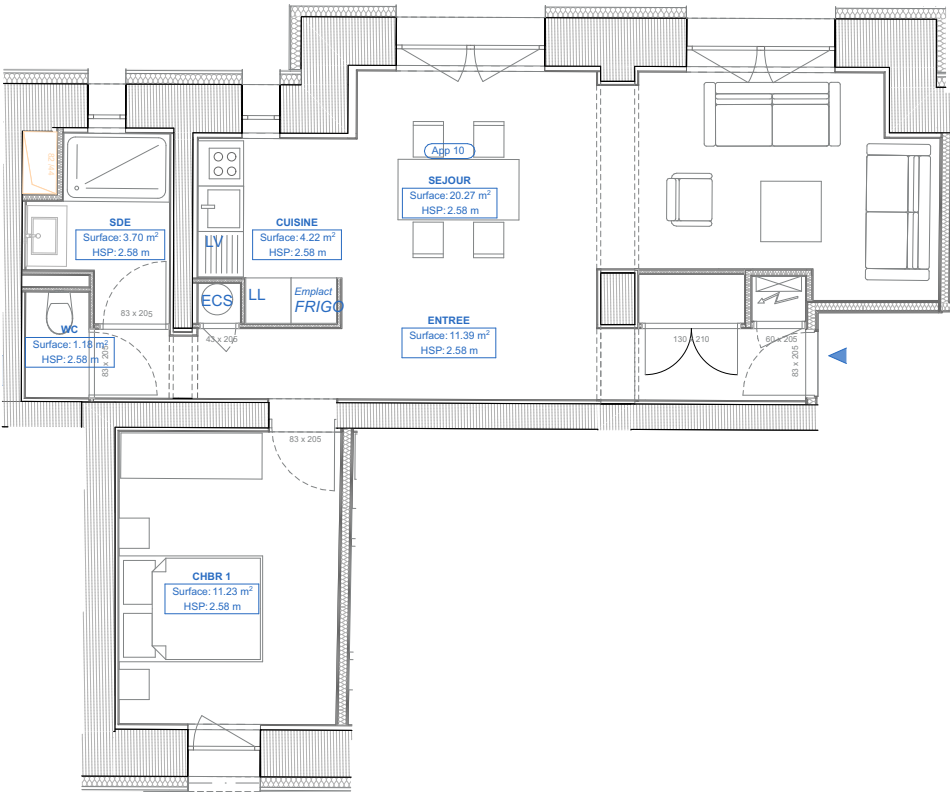
1er étage 1:100
