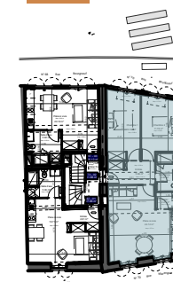
PLAN DE NIVEAU- R+1
