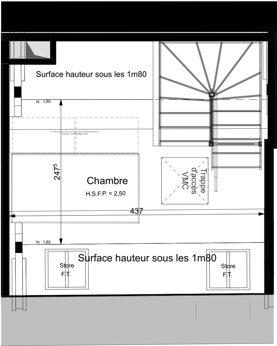
1er étage Premier niveau
