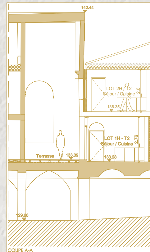
Plan coupe du lot 2H
