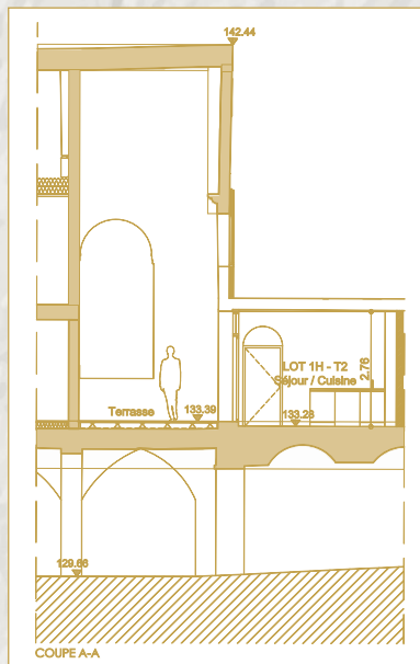
Plan coupe du lot 1H
