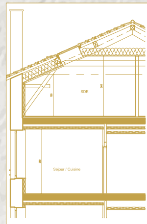
Plan de coupe du lot 2/3C
