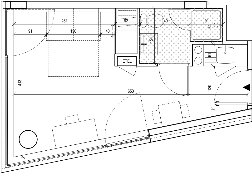
PLAN DU STUDIO (1:50) (côtes en centimètres) L'aménagement intérieur est susceptible de modifications.
