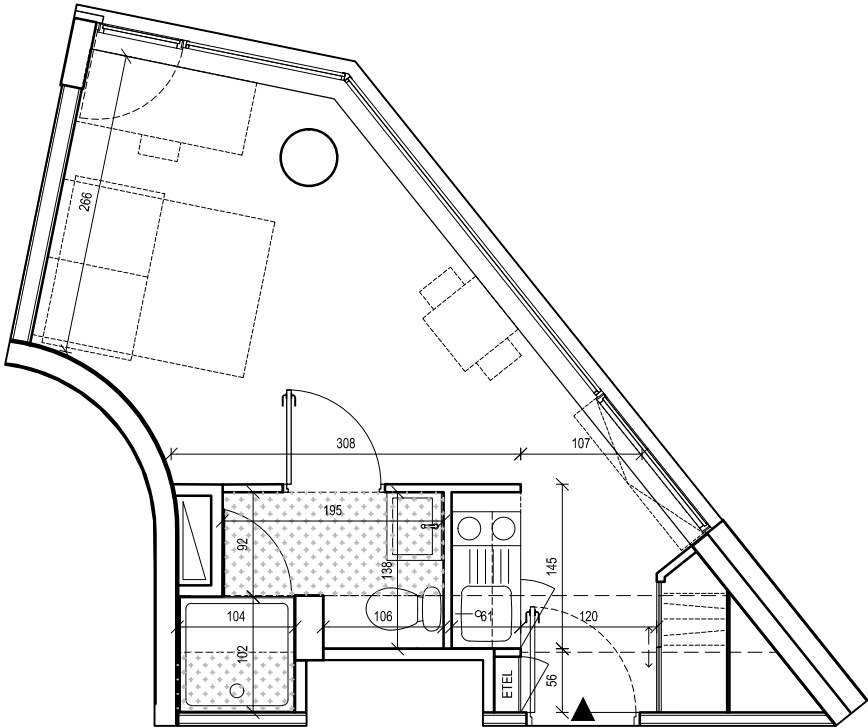
PLAN DU STUDIO (1:50) (côtes en centimètres) L'aménagement intérieur est susceptible de modifications.
