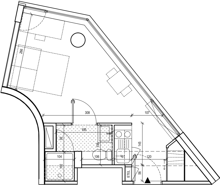
PLAN DU STUDIO (1:50) (côtes en centimètres) L'aménagement intérieur est susceptible de modifications.
