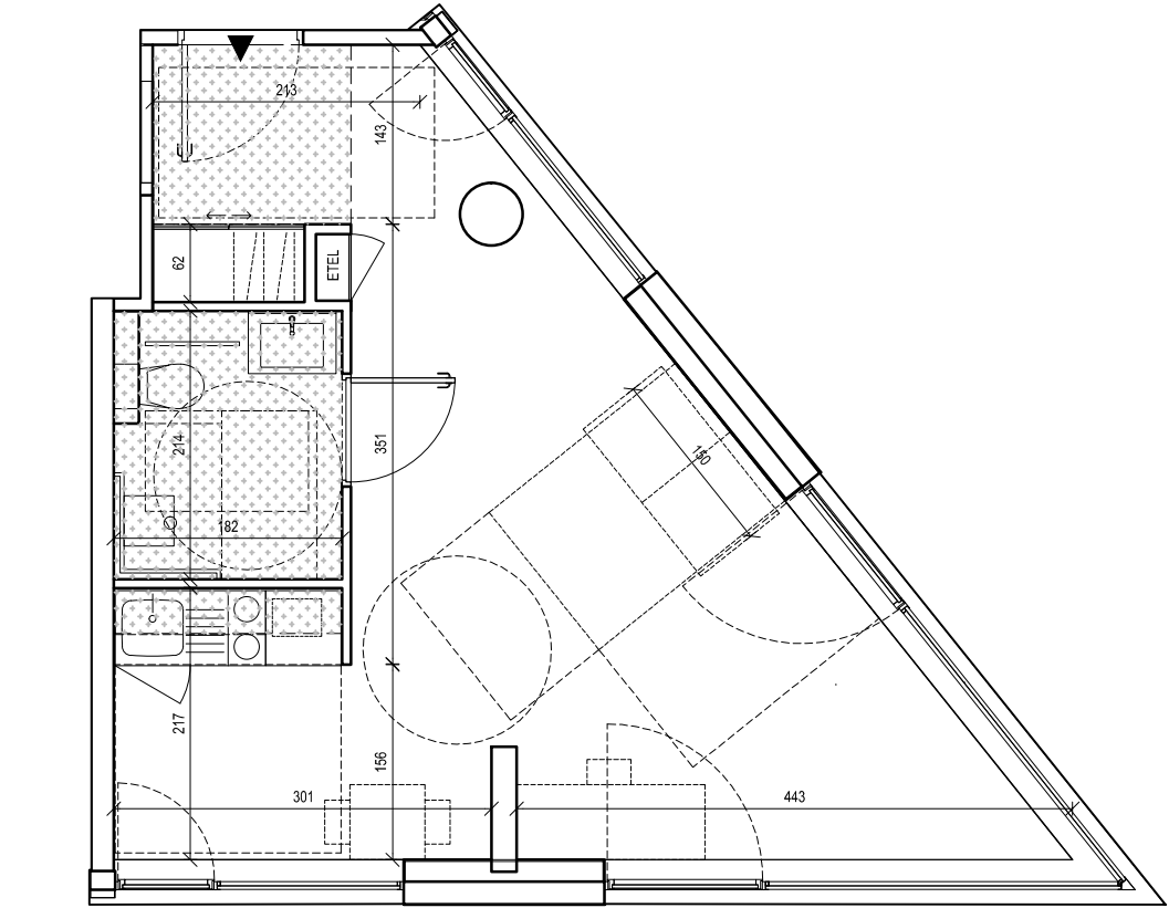
PLAN DU STUDIO (1:50) (côtes en centimètres) L'aménagement intérieur est susceptible de modifications.
