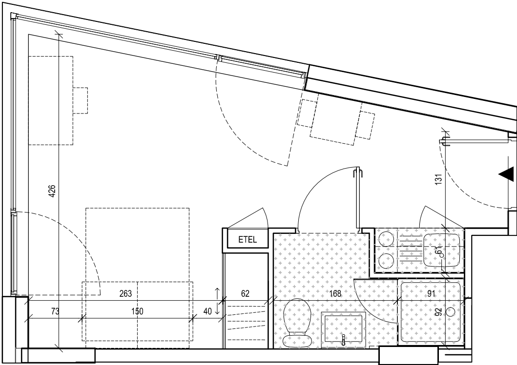
PLAN DU STUDIO (1:50) (côtes en centimètres) L'aménagement intérieur est susceptible de modifications.
