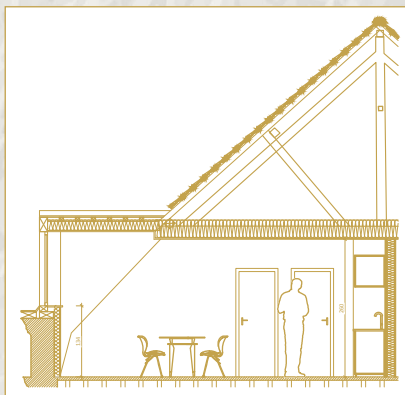
Plan coupe du lot 3B
