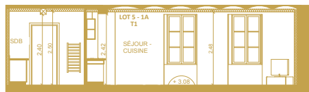
COUPE
