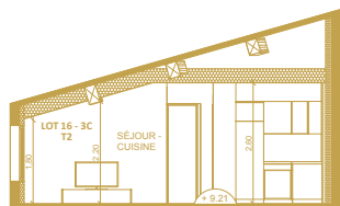
COUPE AA
