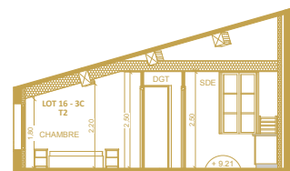
COUPE BB
