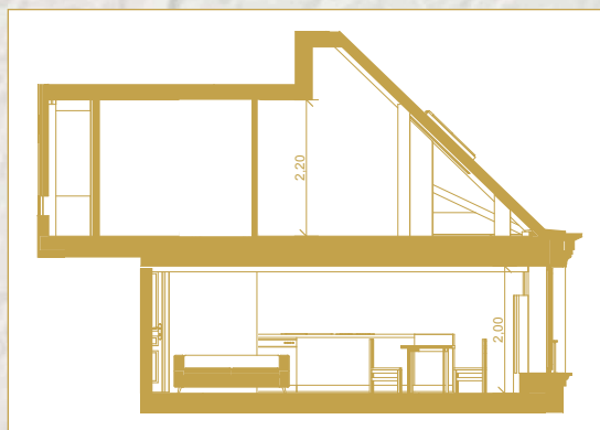
Plan coupe du lot 2/3G
