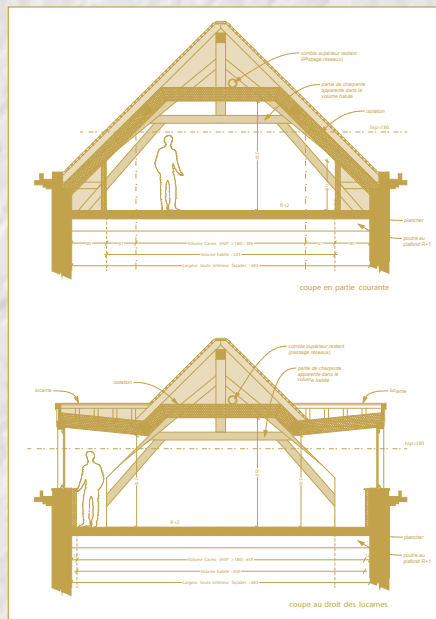
Plan coupe du lot 1/2L
