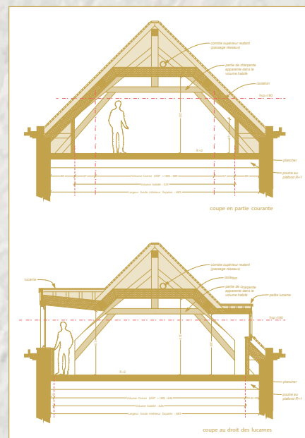
Plan coupe du lot 2B
