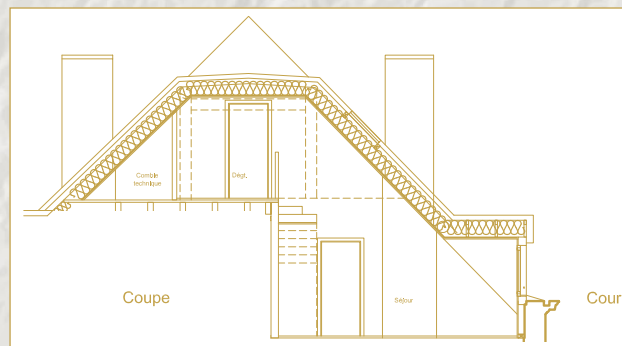
Plan de coupe du lot 4-5C
