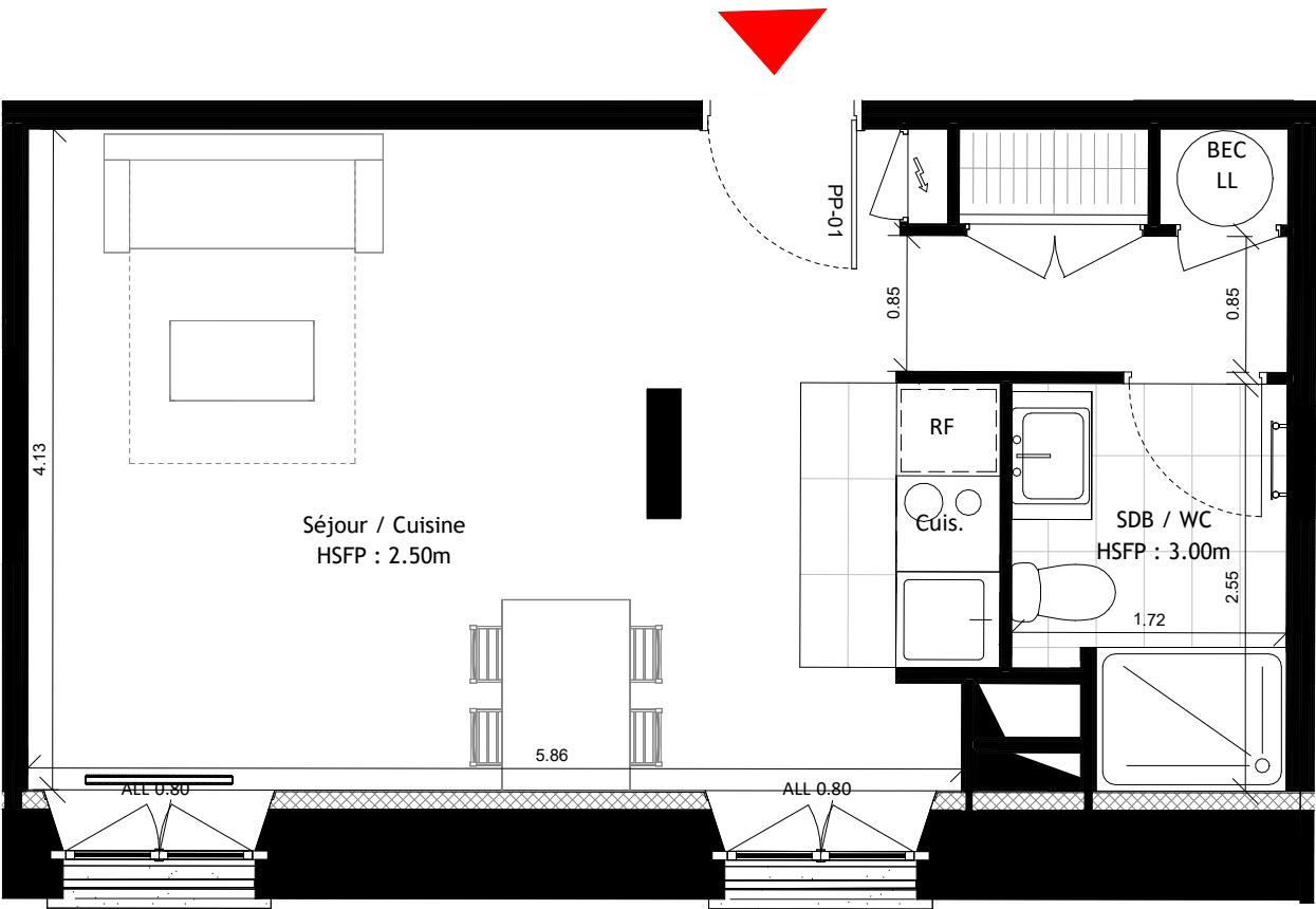
Logement C23B Type T1
